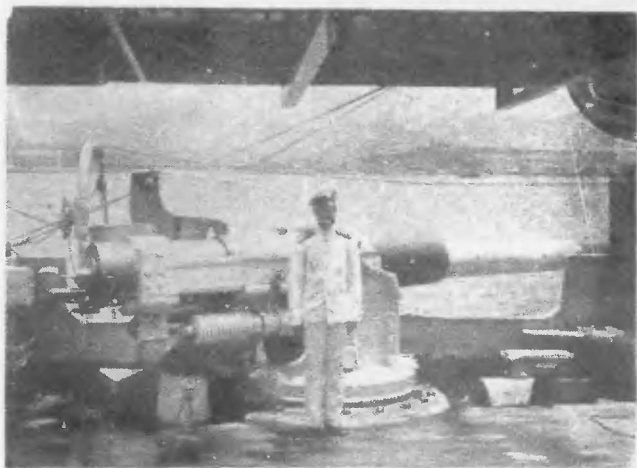
6-ти дюймовое орудіе на «Варягъ».
